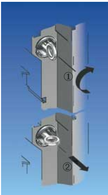
Монтаж шкафа в полую стену с помощью набора UZ 90:
